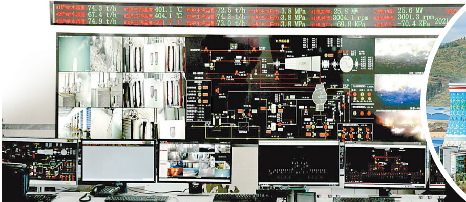
五华垃圾发电厂中控室
