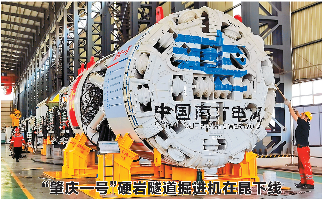
近日,水电十四局参与研制的硬岩隧道掘进机(TBM)“肇庆一号”在昆明下线,标志着国产高端装备技术应用用于抽水蓄能电站建设取得新突破。 “肇庆一号”TBM开挖直径为3.53米,总长约52米,整机总重约220吨,掘进距离约5000米。该TBM专门针对广东肇庆抽水蓄能电站自排排水洞小洞径、长距拖、独头掘进等难题研制,具备超小半径转弯,搭载整机长距离
